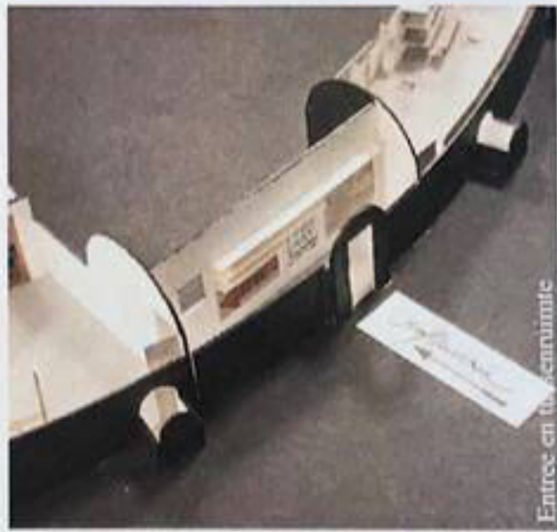
Totaaloverzicht caponniere Wilcke in maquettevorm
